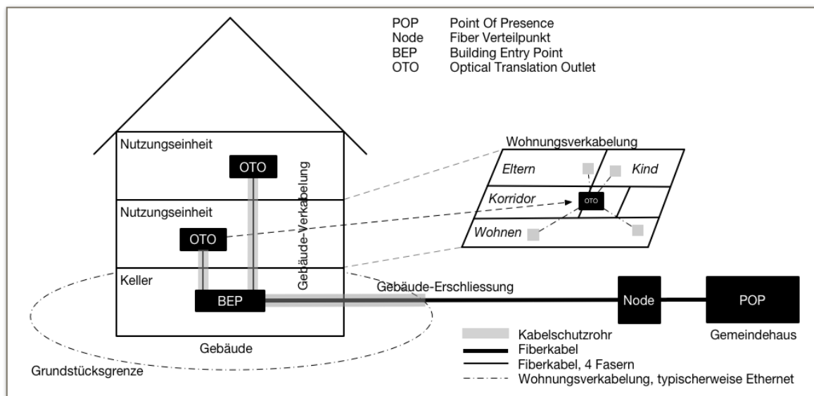
FTTH (Fiber To The Home) Gebäuderverkabelung, Prinzipschema
